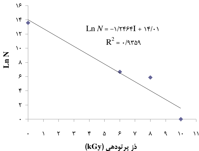
شکل ۱. نمودار پابندگی-دُز میکروارگانسیم‌های آویشن پس از پرتودهی با اشعه گاما.
