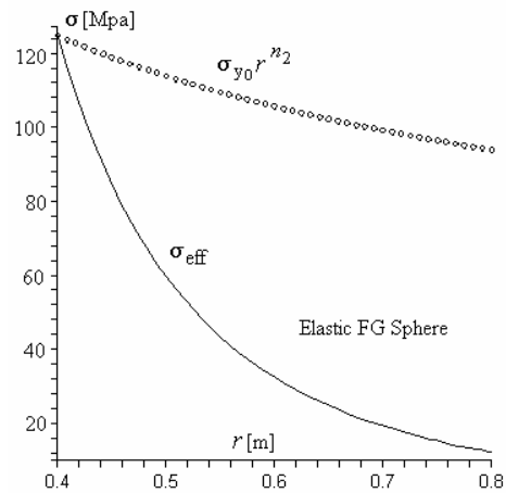
شکل (۲): تنش موثر کره الاستیک FG در آستانه تسلیم
