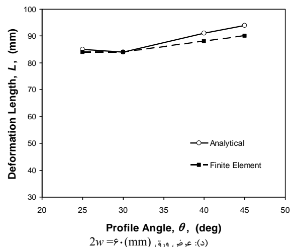
شکل (۸): اثر افزایش زاویه ی پروفیل بر روی طول تغییر شکل، به ازای عرض ورق ثابت، برای فرایند نمونه ی مورد بررسی.
