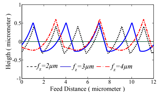
شکل (۷): زبری سطح ایجاد شده با پیشروی های متفاوت ( r_e = 3 \mu\text{m} )
