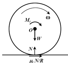
شکل (۷): نمایش نیروی های وارده به چرخ.
