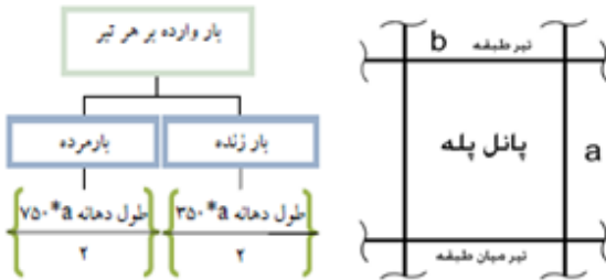
شکل ۲- پانل پله در مدل‌سازی (حالت ۱)
