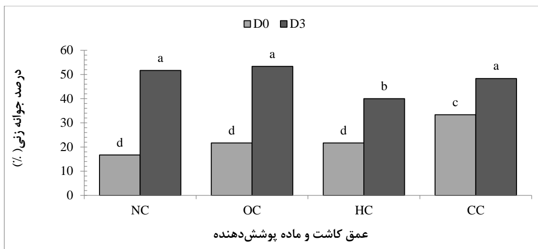
شکل ۲- اثر متقابل نوع ماده پوشش دهنده (NC، OC، HC و CC) در عمق کاشت سطحی (D0) و عمق کاشت سه برابر قطر بذر (D3) بر درصد جوانه زنی گونه خلر
