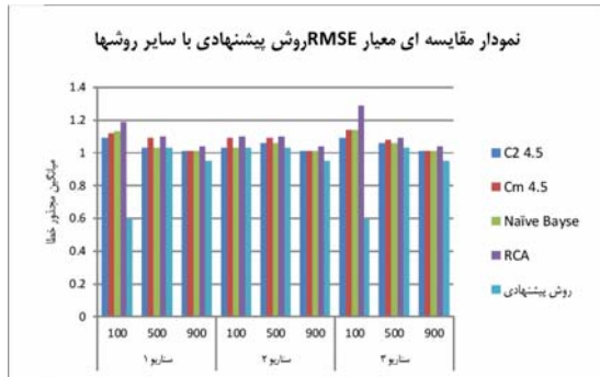
شکل ۵- مقادیر مربوط به RMSE برای تعداد کاربران
