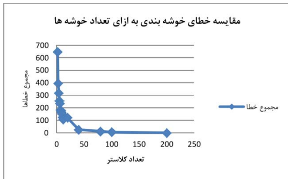
شکل ۲- مقایسه مجموع مربعات خطا خوشه بندی به ازای تعداد k های مختلف
