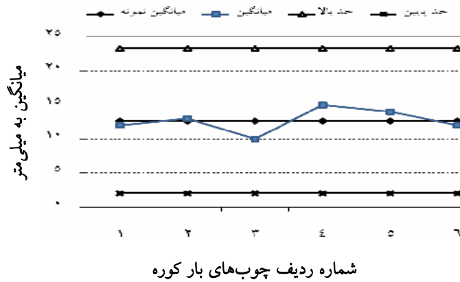
شکل 5- نمودار C برای تعداد عیوب ایجاد شده در مرحله دوم
