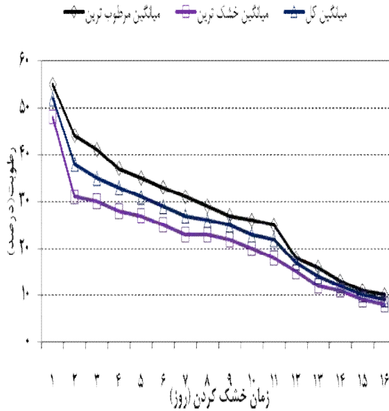
شکل 2- کاهش رطوبت چوب‌های بار کوره طی زمان در مرحله دوم
