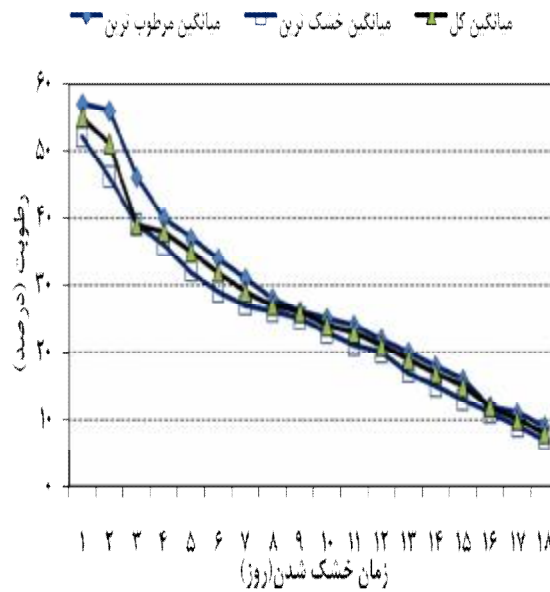
شکل 1- کاهش رطوبت چوب‌های بار کوره طی زمان در مرحله اول
