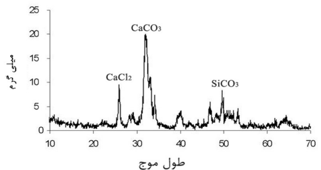
نمودار ۴: آزمون XRD تولید کربنات کلسیم در محیط مایع جدایه اسپوروسارسینا پاسترویی KT862894
