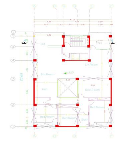
شکل ۱- پلان معماری ساختمان
