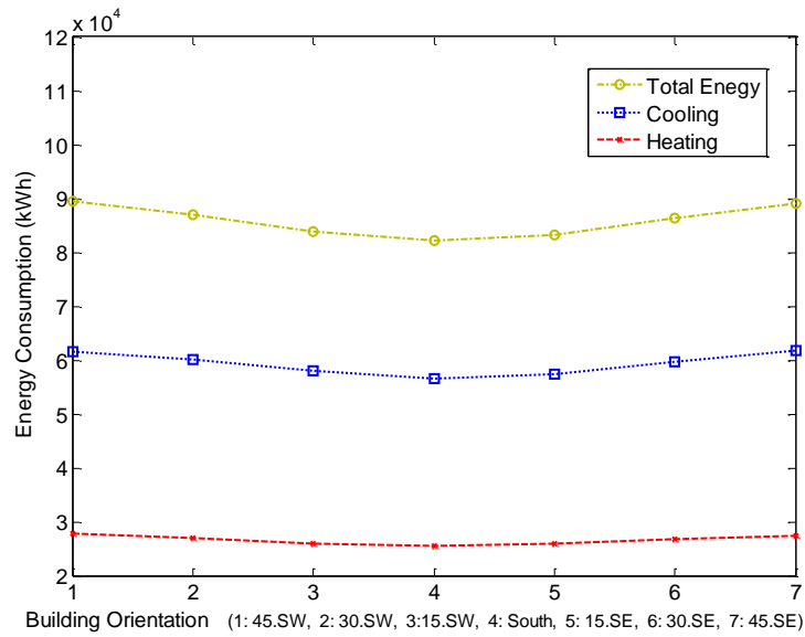
شکل ۷. انرژی مصرفی سالانه نمونه موردی با شاخص تناسب ۱:۲ در جهت گیری های پیشنهادی در شهر رشت
