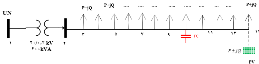
شکل (۴): آرایش فیدر توزیع ۱۴ باسه مورد مطالعه با مکان احتمالی نصب خازن و PV Figure (4): Topology of feeder distribution 14-bus with possible location installation of PV and FC
