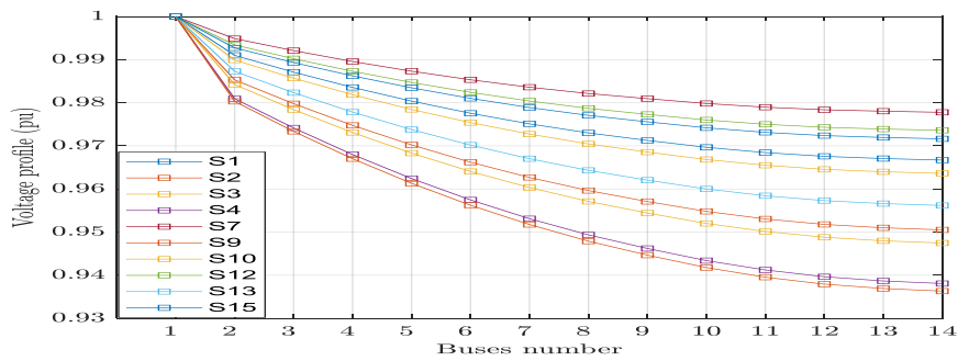
شکل (۶): دامنه ولتاژ باس‌ها و سناریوهای مختلف در حالت جبران‌سازی با خازن برای شبکه ۱۴ باسه در حالت ۲ Figure (6): Voltage profile of different busses with 22-scenarios in mode 2 without compensation for 14-bus network
