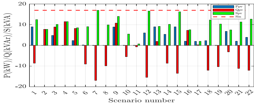
(الف) توان تولید شده با PV نصب شده در باس ۱۴ با حضور FC و قابلیت اینورتر با اضافه ظرفیت ۱۷ کیلوولت-آمپر
