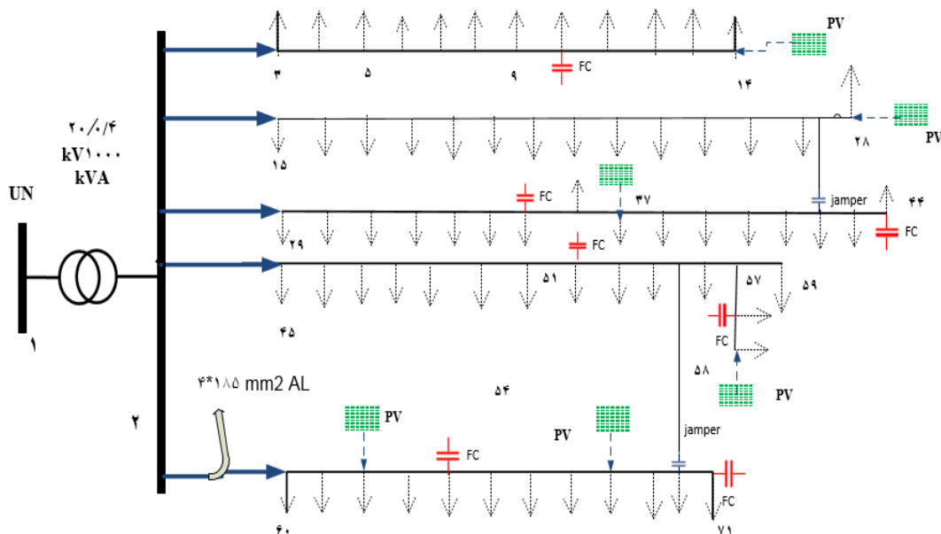
شکل (۱۳): آرایش شبکه توزیع ۷۱ باسه مورد مطالعه با مکان‌های احتمالی نصب PV و FC Figure (13): Arrangement of feeder distribution 71-bus with possible location installation of PV and FC
