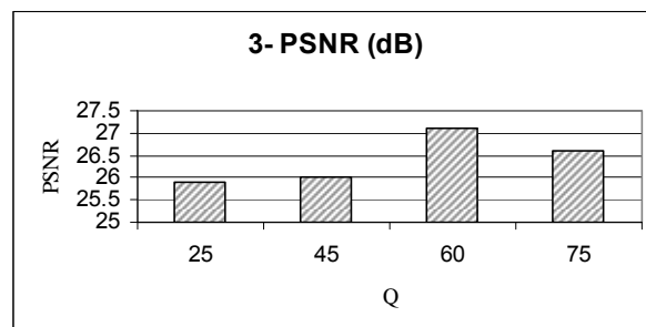
شکل ۱۸- نتایج PSNR (MDC-Line-with zero) با ۱/۵٪ نویز و Qهای مختلف با تصویر Lena
