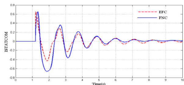
شکل ۱۱- جریان STATCOM
