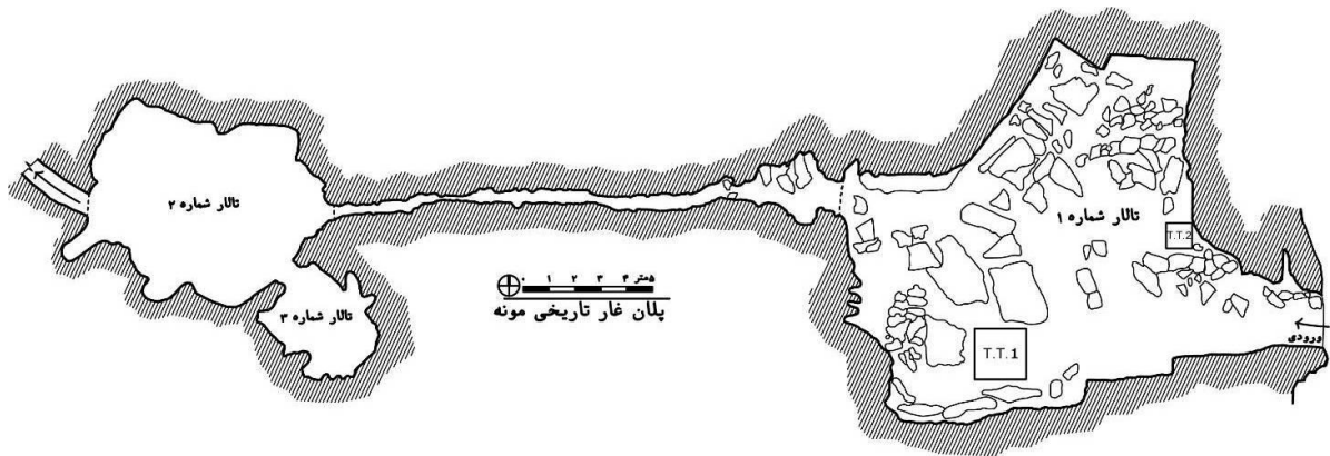
شکل ۴: برش عمودی از غار نمونه و تالارهای موجود در آن
