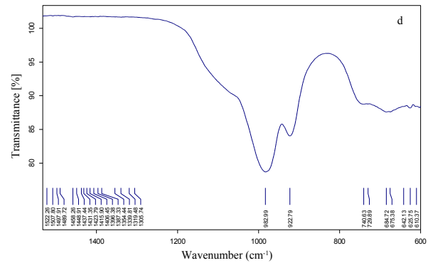
شکل ۳ طیف‌های FT-IR نمونه‌های تهیه شده (a) NaX (b) TiX (c) NiX (d) CoX (e) ZnX (f) NiTiX (g) CoTiX (h) ZnTiX
