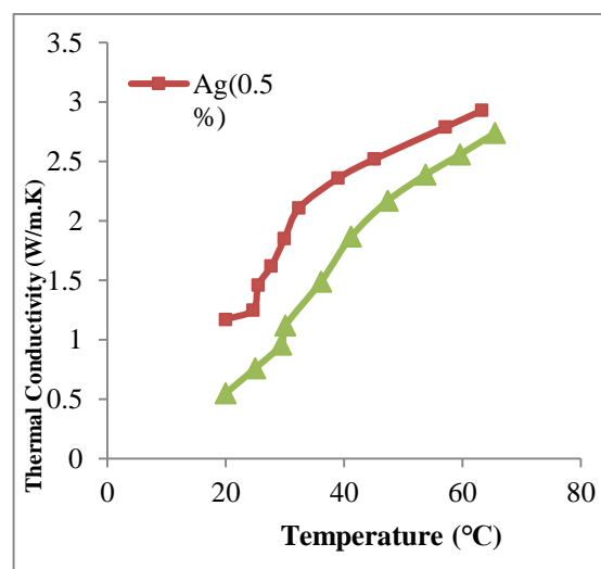
شکل (۹): مقایسه بین هدایت حرارتی نانوسیال حاوی نانومیله های نقره و نانومیله های مس در غلظت ۰/۵ درصد وزنی
