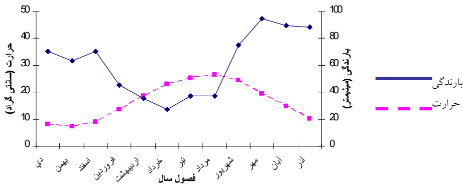
شکل ۲- منحنی آمپروترمیک منطقه مورد مطالعه در فاصله سال‌های ۱۳۶۶-۱۳۸۶
