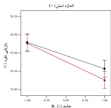
شکل ۴ تأثیر متقابل عامل‌ها در آزمایش‌های فروشویی سیانیدی بر بازبایی نقره
