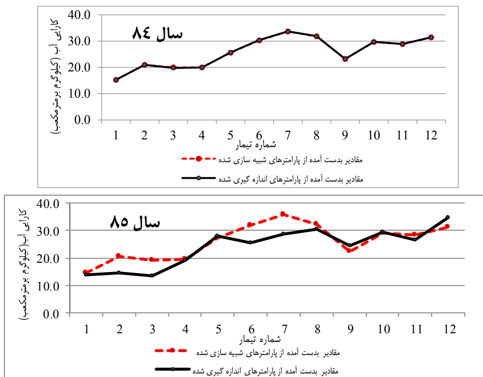
شکل ۲- مقایسه مقادیر کارایی مصرف آب بدست آمده از پارامترهای اندازه‌گیری و شبیه‌سازی در مراحل واسنجی و اعتبارسنجی
