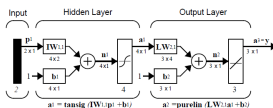
شکل ۳: شبکه عصبی پرسپترون چند لایه
